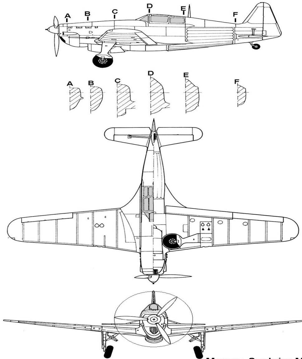
Morane-Saulnier MS-410
